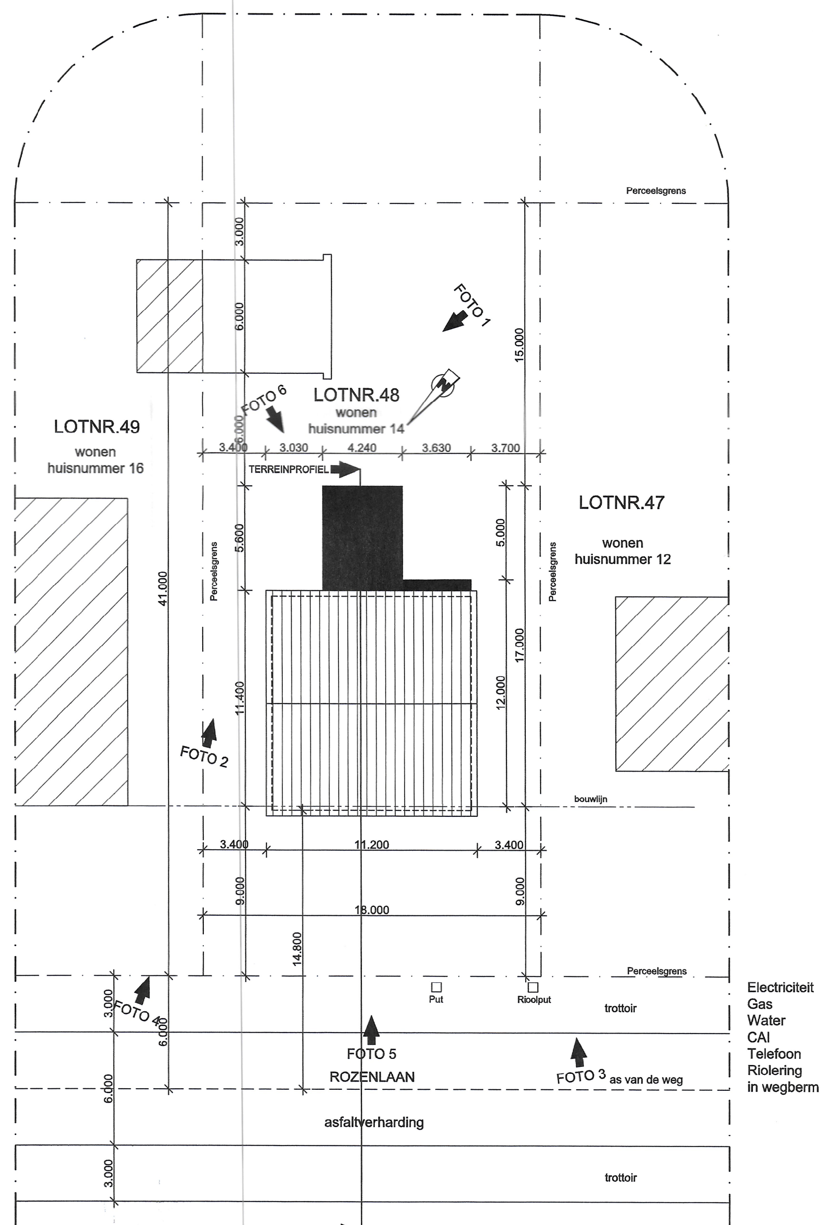
INPLANTINGSPLAN 1 : 200
