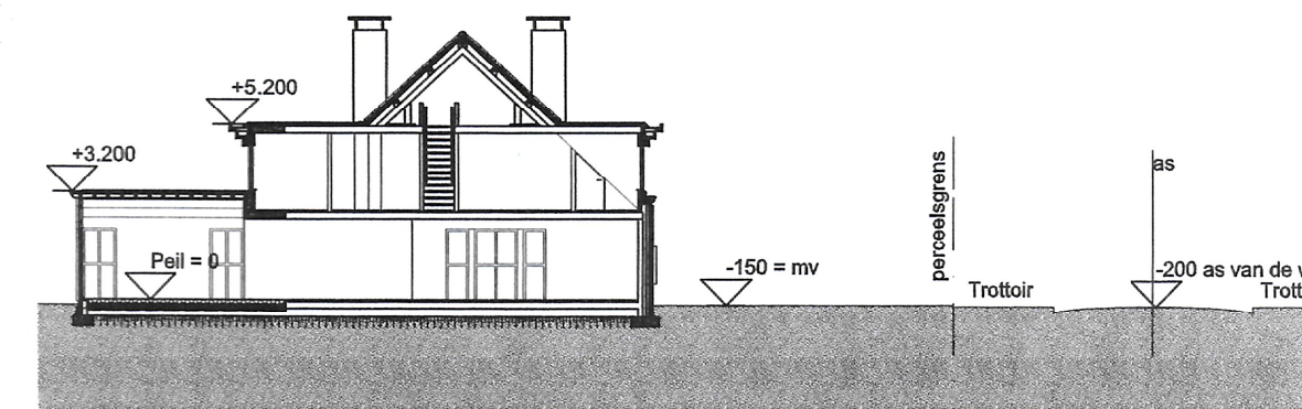
TERREINPROFIEL 1 : 250
